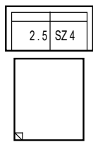
2.5SZ4 W:198 x D:100-209 x H:87cm
