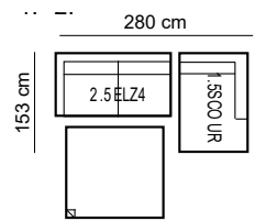
2.5ELZ4 + 1.5SCOUR W:280 x D:153/209 x H:87cm
